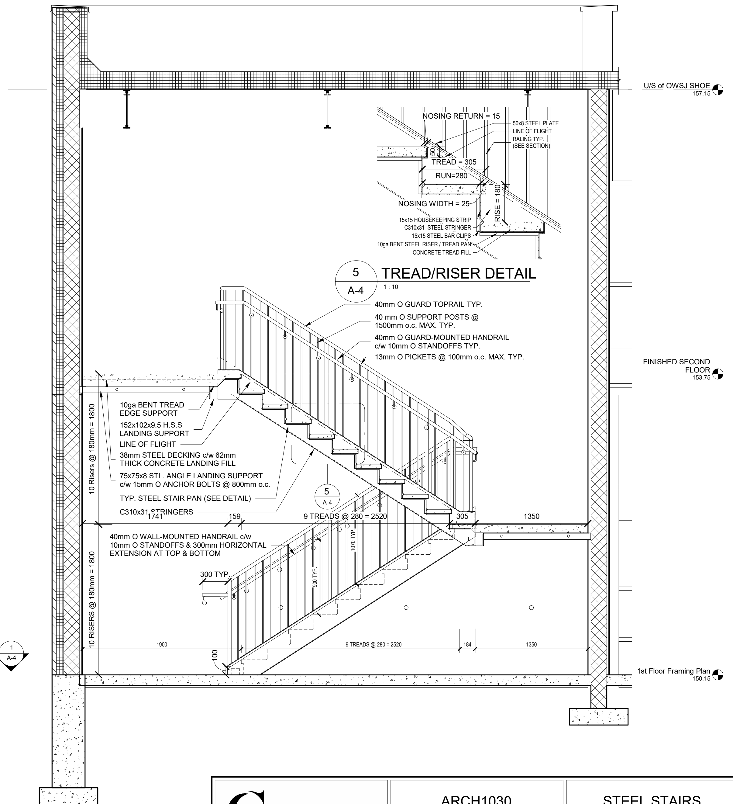
1 STAIR SECTION 1:25 A-4
